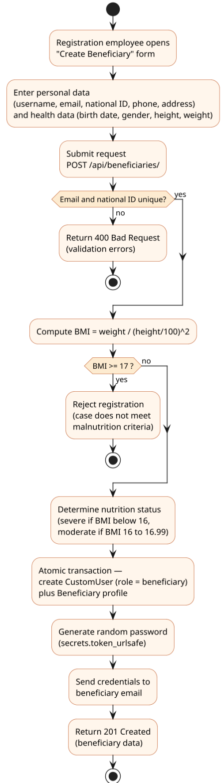
الشكل (3-5) مخطط النشاط لعملية تسجيل مستفيد جديد
