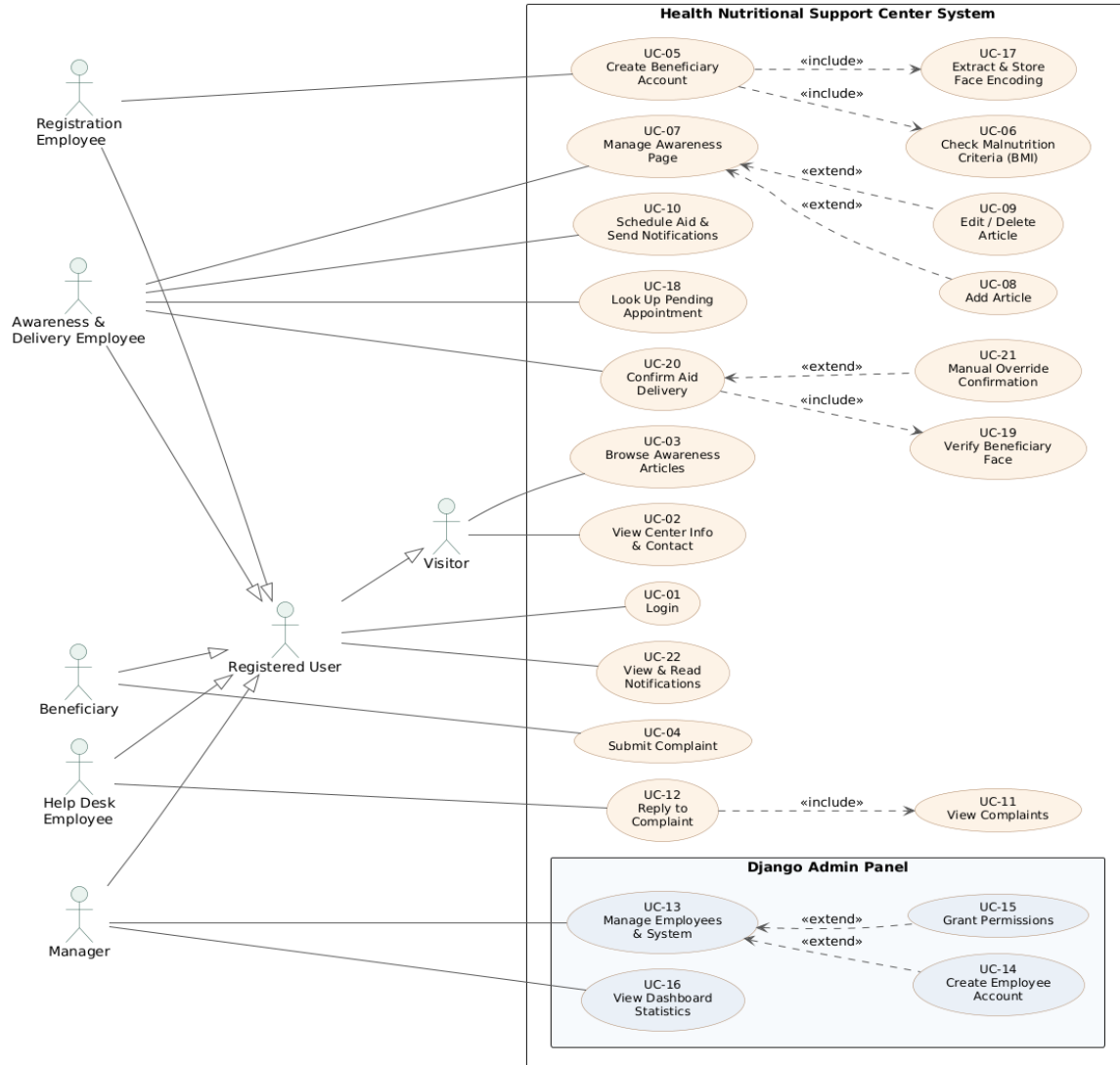
الشكل (1-2) مخطط حالات الاستخدام العام للنظام
