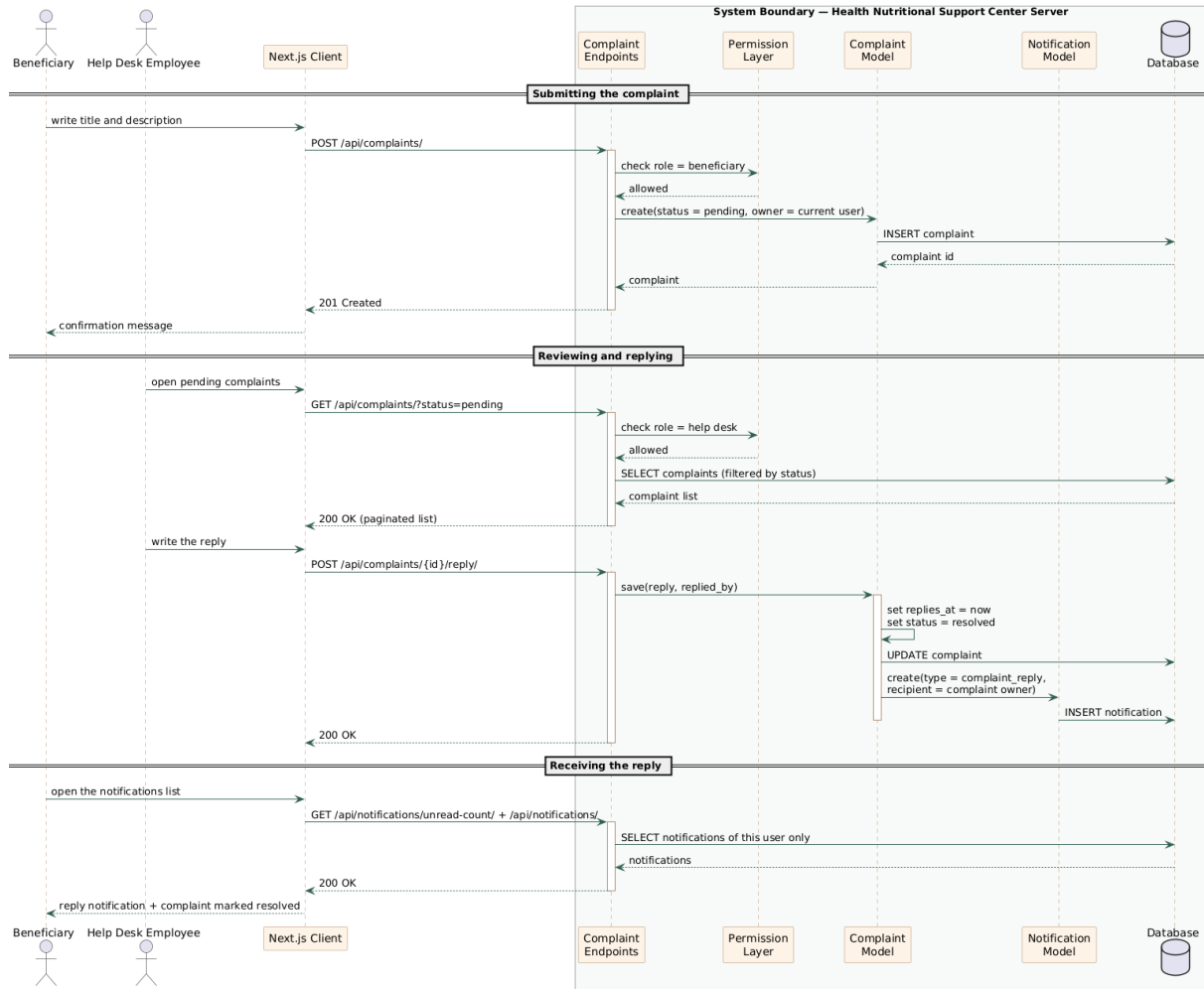
الشكل (3-4) مخطط التسلسل لدورة الشكوى والرد عليها
