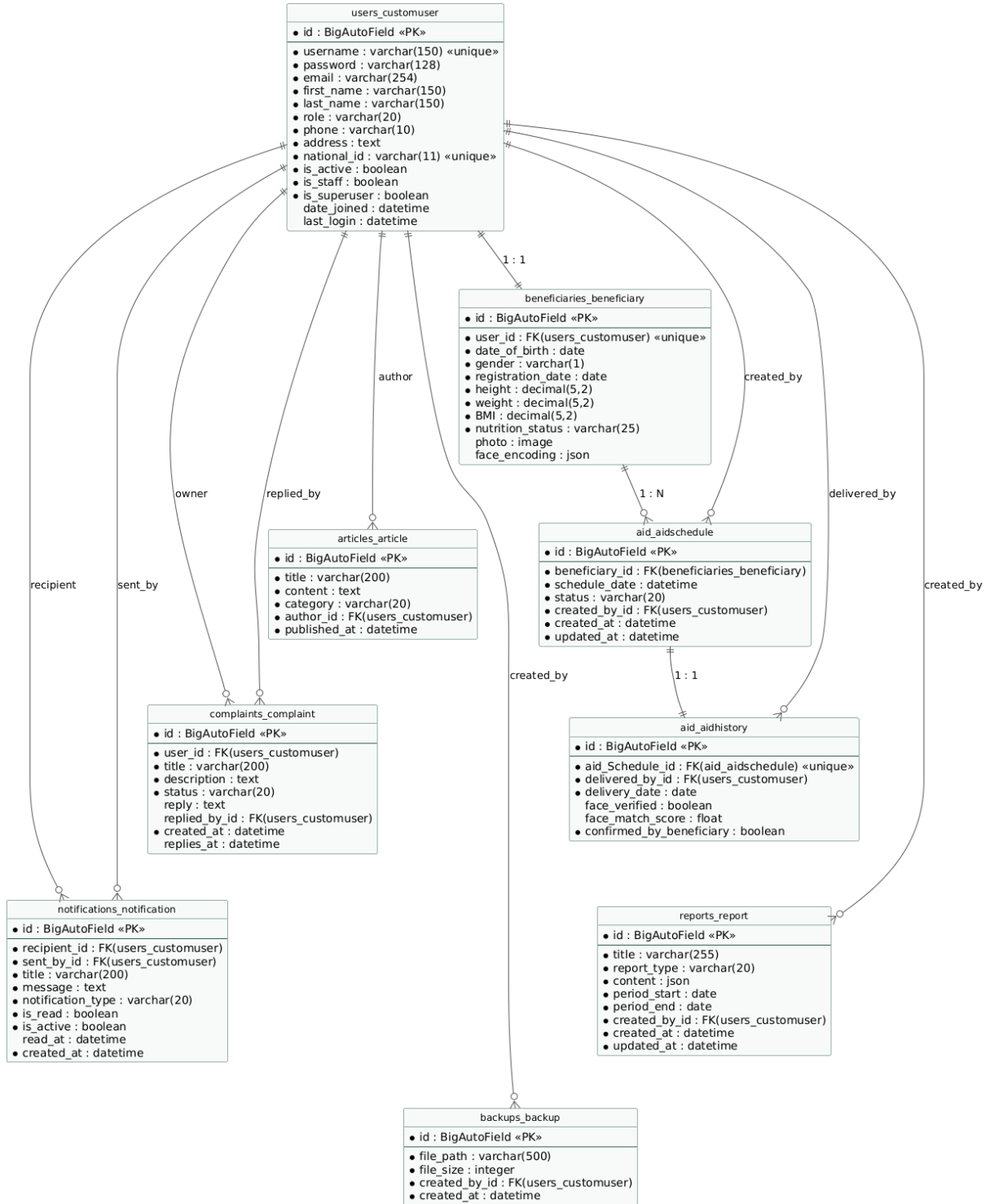
الشكل (2-3) مخطط الكيانات والعلاقات لقاعدة بيانات النظام
