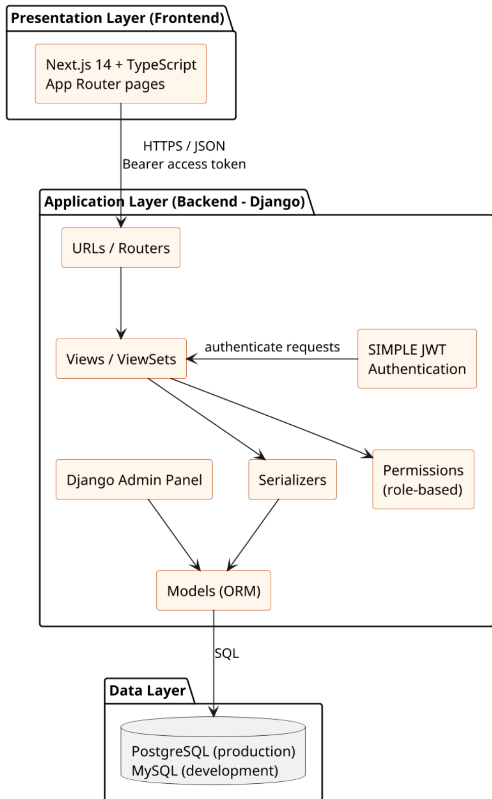
الشكل (1-3) المعمارية العامة للنظام وطبقاتها
