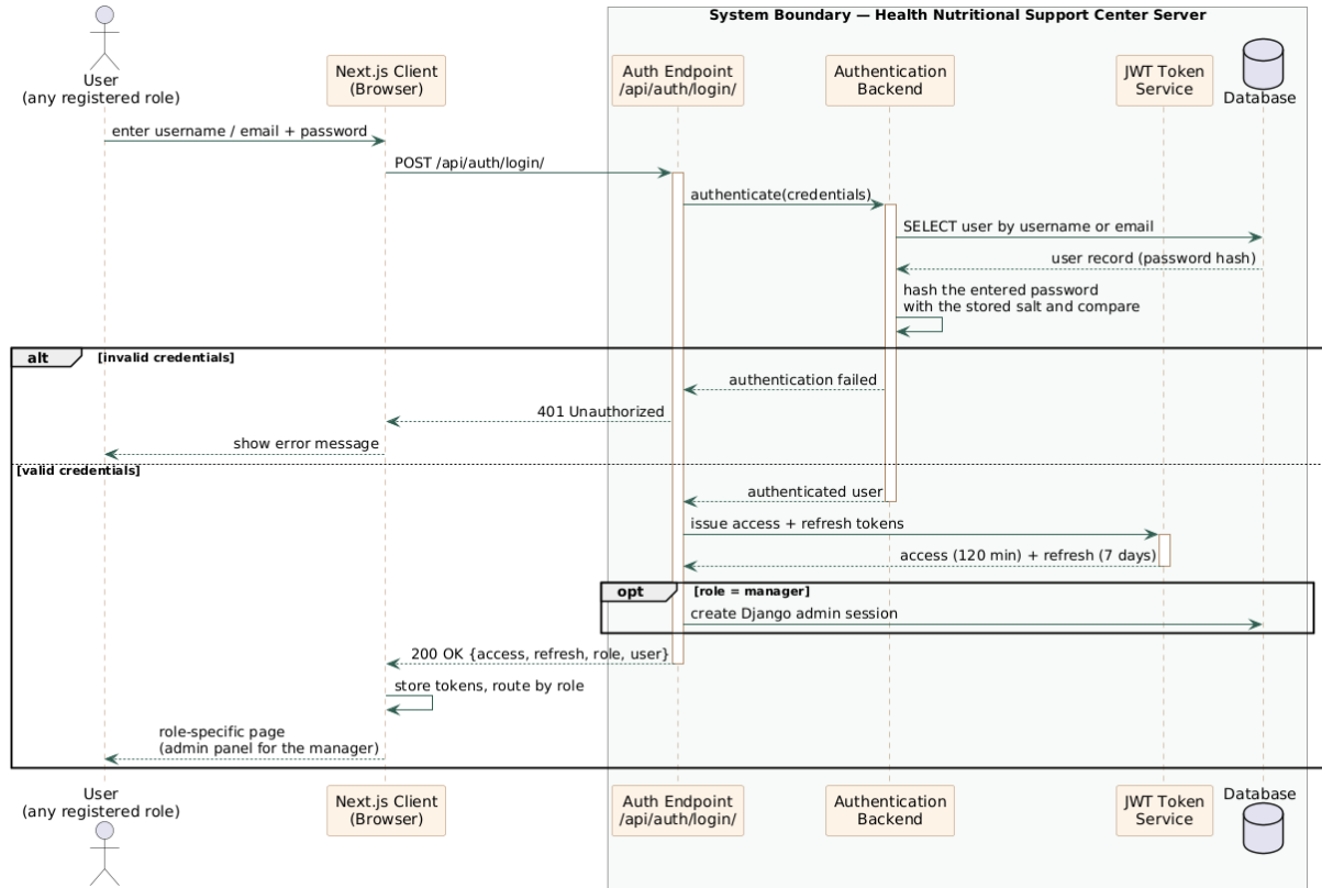
الشكل (3-3) مخطط التسلسل لعملية تسجيل الدخول
