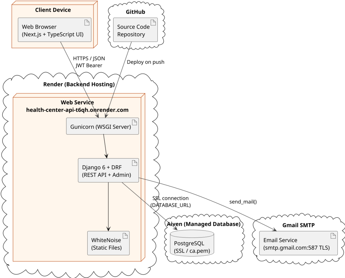
الشكل (6-3) مخطط النشر وتوزع مكونات النظام
