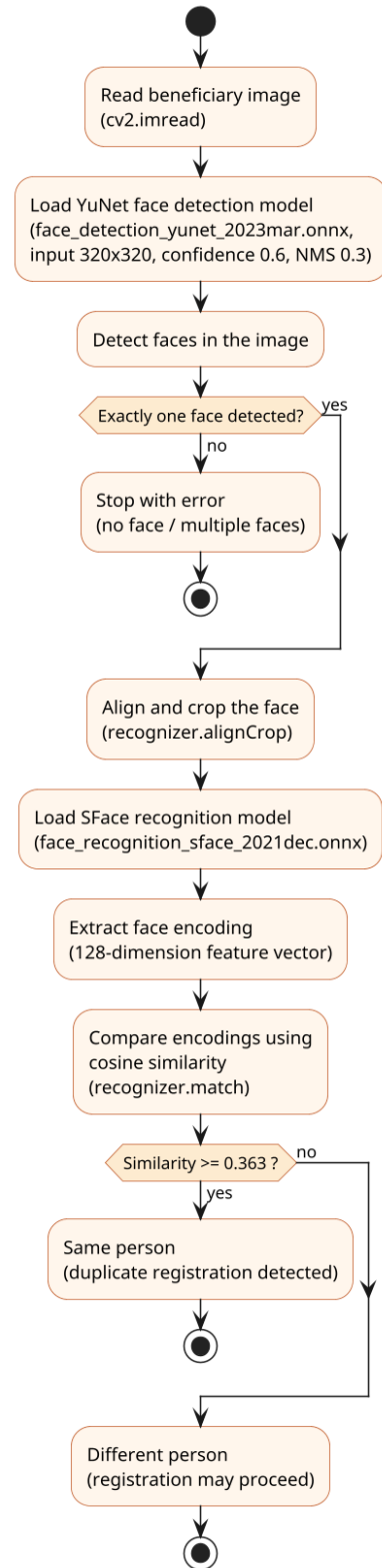
الشكل (4-1) التدفق التصميمي لميزة التحقق من الوجه
